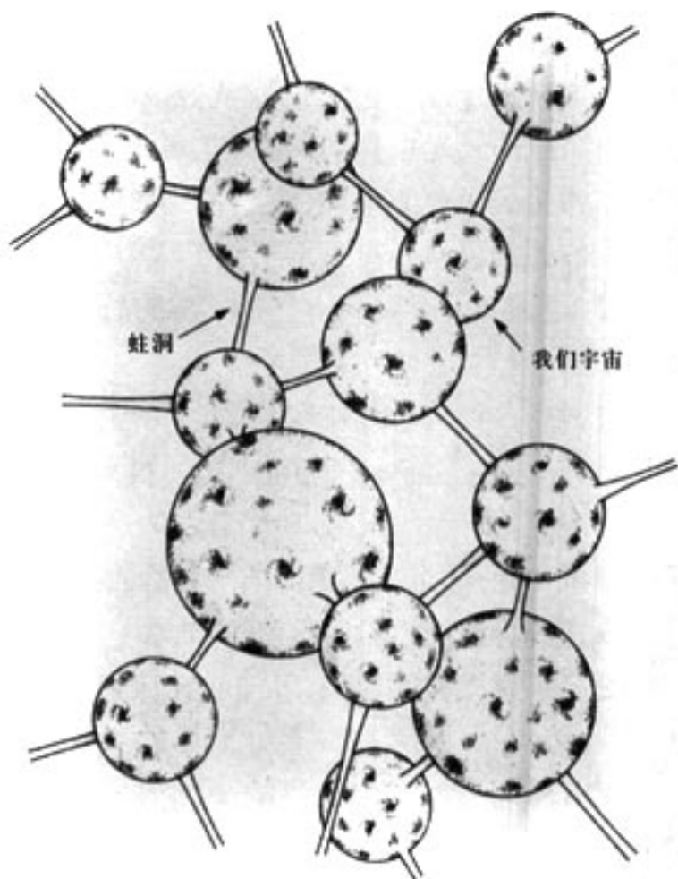
我们宇宙或许是无数个平行宇宙中的一个。每一个宇宙通过无穷多的蛙洞（连通两个时空域的隧道）跟其他宇宙相连。在这些蛙洞之间旅行是可能的，但可能性又微乎其微。
